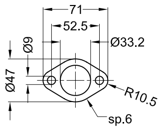
Flangia "43A"
