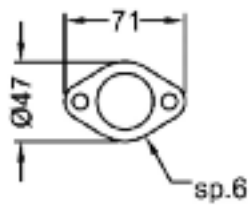
Vista "B" Flangia "43A"
