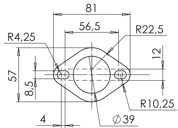
Flange 25b
